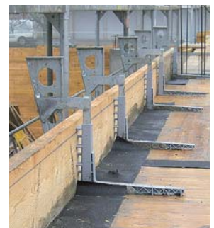
Seitenabschlag
